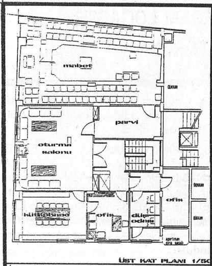
ÜST KAT PLANI 1/50
