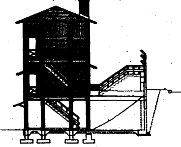
SAĞ CEPHE
